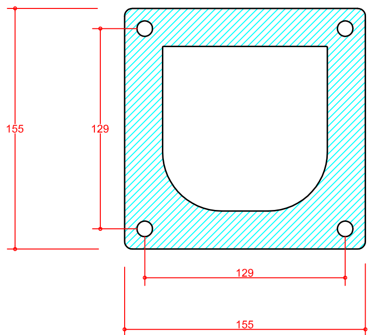
Pfostenboden mit Flansch
