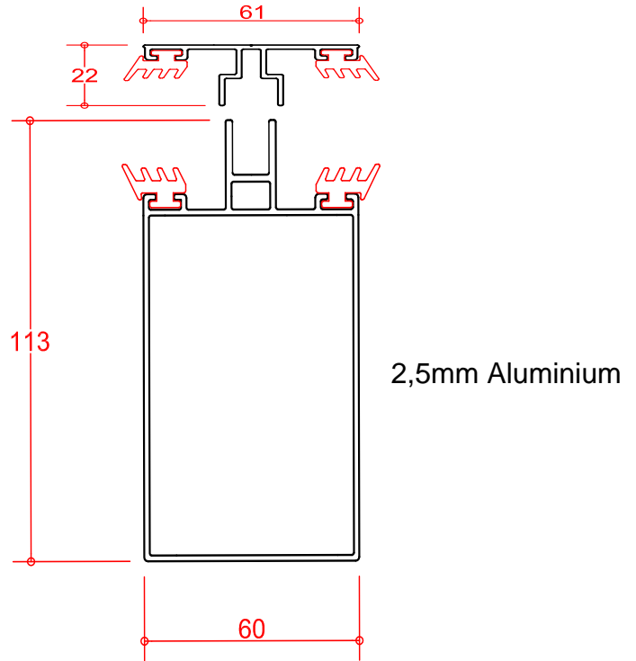
Pfostenboden mit Flansch
